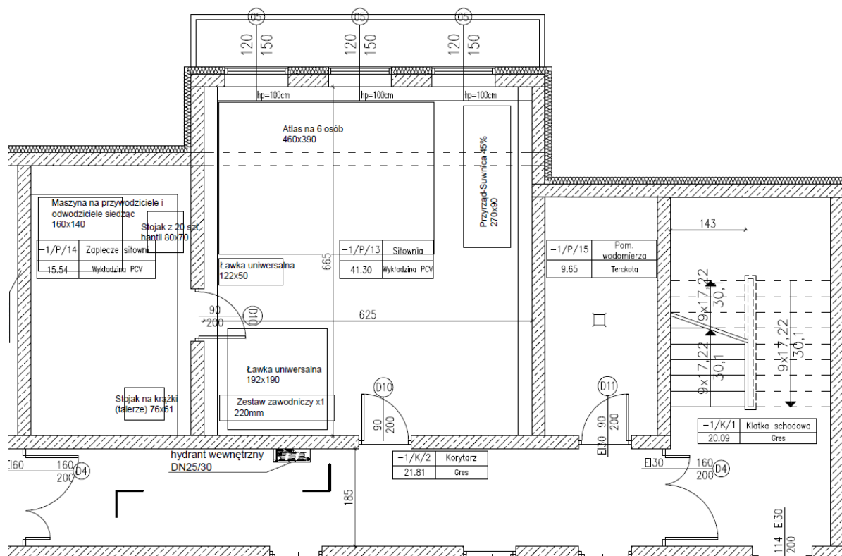
rysunek nr 1. Rzut pomieszczeń siłowni wraz z rozmieszczeniem sprzętu będącego przedmiotem zamówienia.
